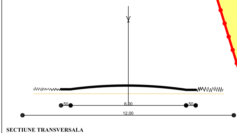
SECTIUNE TRANSVERSALA
